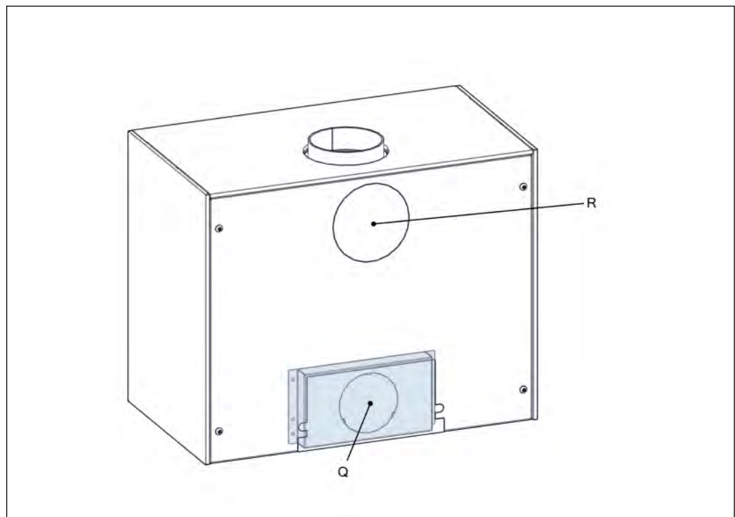
Abbildung 3. Rückansicht der BOX 20 52
