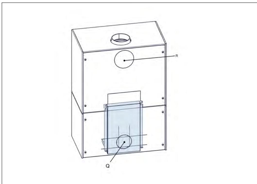
Abbildung 6. Rückansicht der BOX 20 80 mit Holzscheit-Speichermodule
