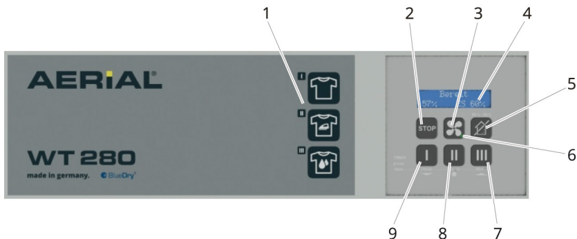
Abb. 4: Bedientableau
