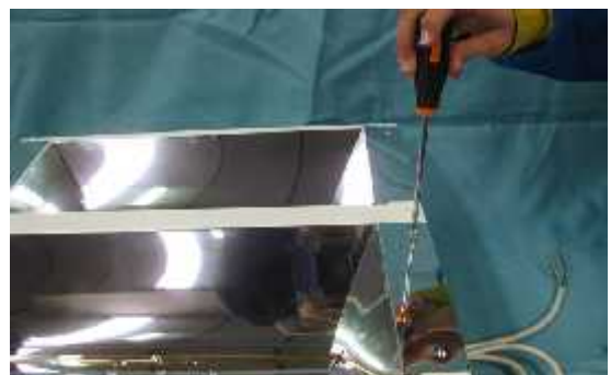
8. ВСТАВЬТЕ БОКОВЫЕ ЧАСТИ РЕФЛЕКТОРА И ЗАКРЕПИТЕ ИХ ВИНТАМИ.
