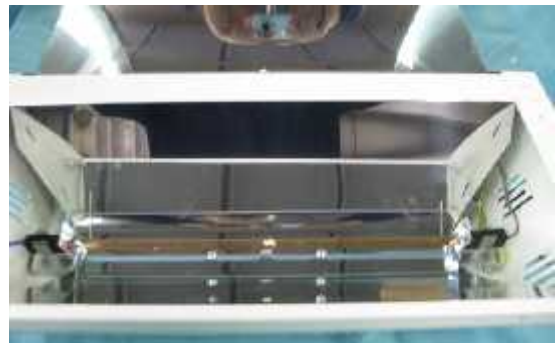
7. КОНЦЫ ЛАМПЫ, ПОКРЫТЫЕ СИЛИКОНОВЫМИ ПРОКЛАДКАМИ, УСТАНОВИТЕ ВНОВЬ В ИЗНАЧАЛЬНОЕ МЕСТО НАХОЖДЕНИЯ, УСТАНОВИВ НА ПРУЖИНЫ.
